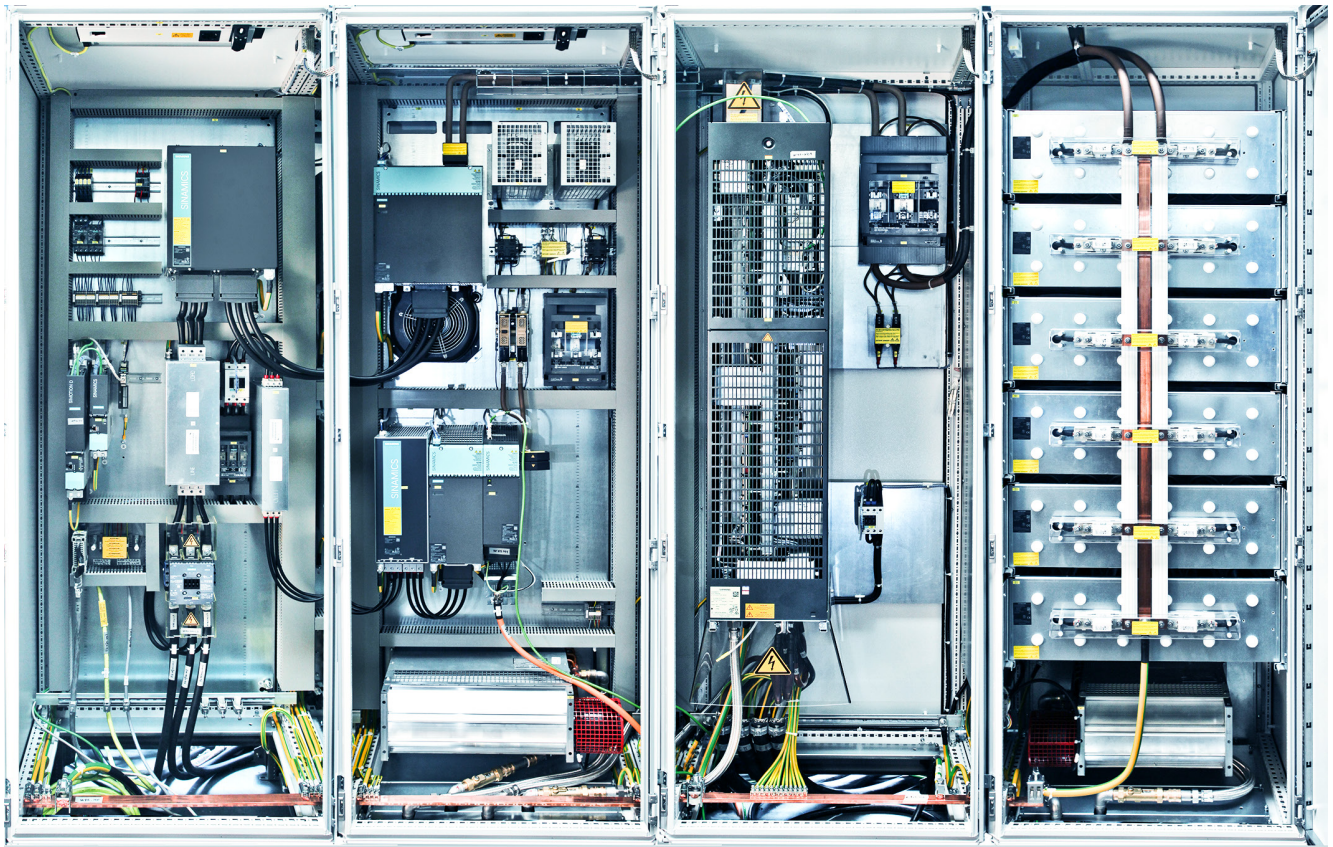
Antriebsschrank einer 3150 kN Servopresse
